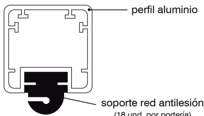
SECCIÓN PERFIL MARCO 80 x 80 mm
